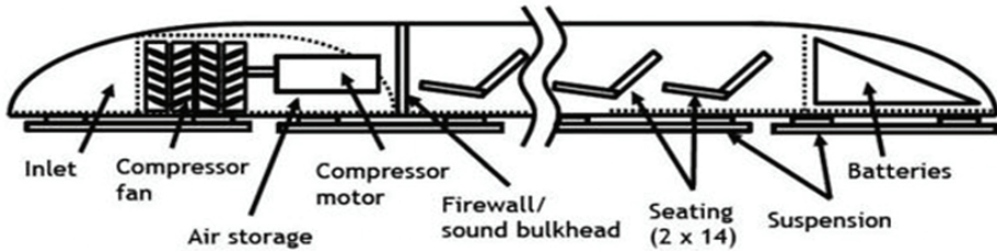
Rys. 4. Schemat kapsuły pasażerskiej
