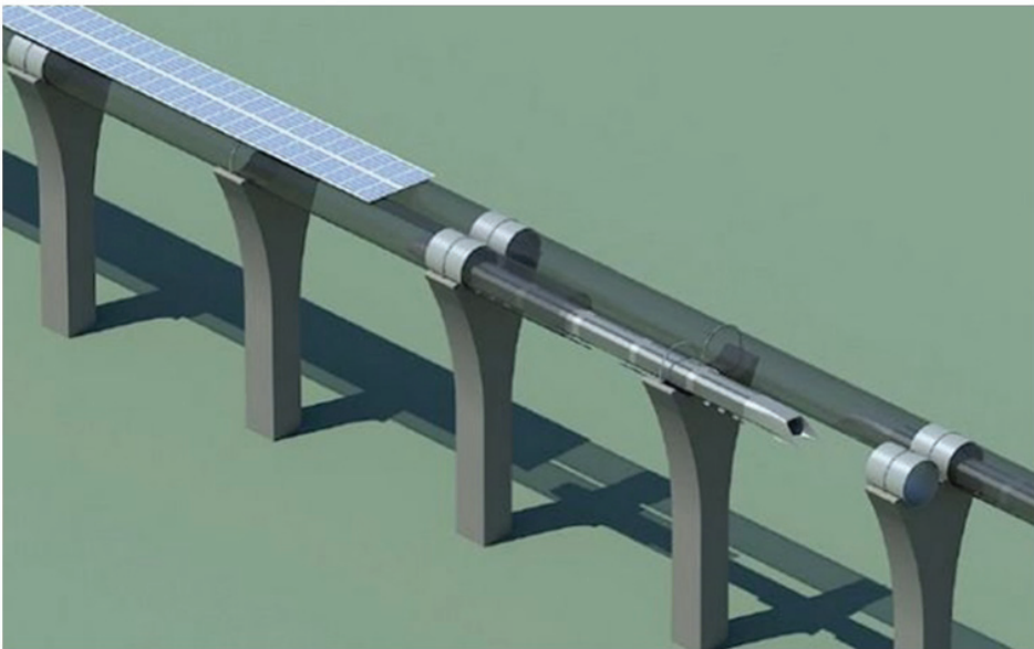
Rys. 5. Trasa Hyperloop One na palach, zasilanie panelami słonecznymi
