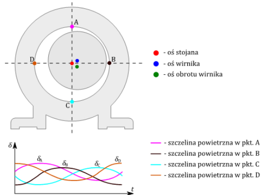
Rys. 3. Ekscentryczność mieszana
