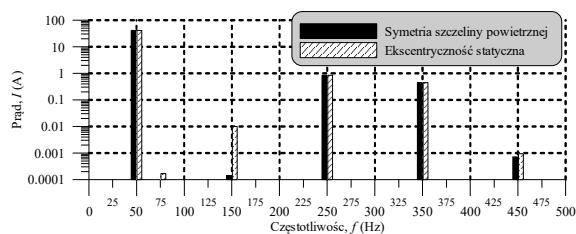
Rys. 6. Widma częstotliwościowe prądu – symulacje komputerowe
