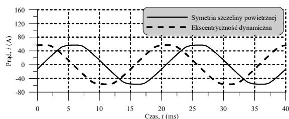
Rys. 7. Przebiegi czasowe prądu – symulacje komputerowe
