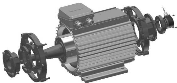
Rys. 10. Generator ze zmodyfikowanymi tarczami łożyskowymi
