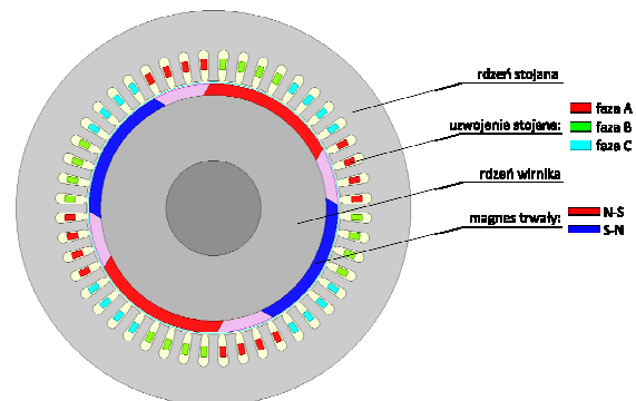
Rys. 4. Model polowo – obwodowy generatora z magnesami trwałymi typu
