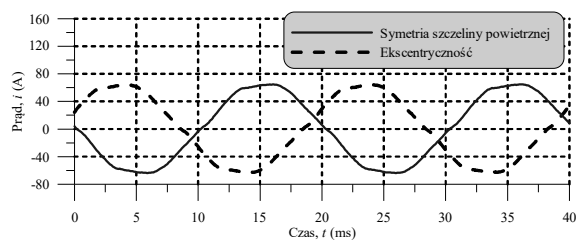
Rys. 11. Przebiegi czasowe prądu – badania laboratoryjne
