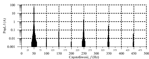
Rys. 12. Widmo częstotliwościowe prądu dla symetrycznej szczeliny powietrznej
