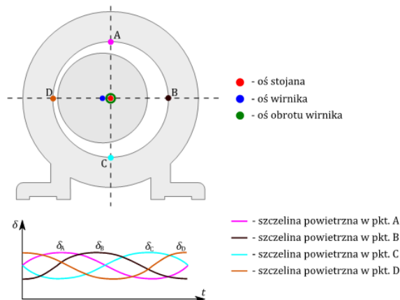
Rys. 2. Ekscentryczność dynamiczna
