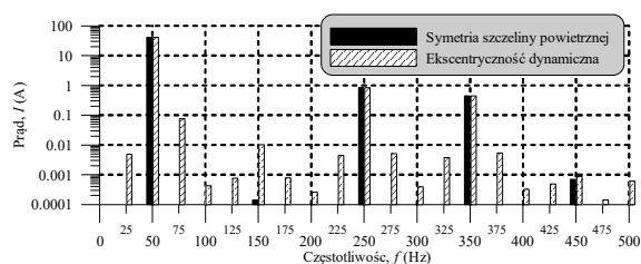
Rys. 8. Widma częstotliwościowe prądu – symulacje komputerowe
