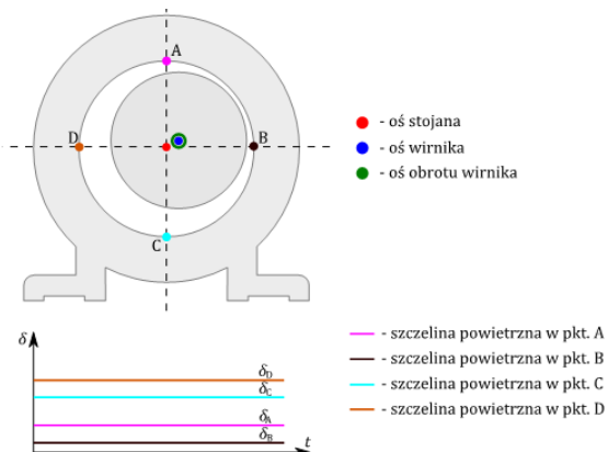
Rys. 1. Ekscentryczność statyczna
