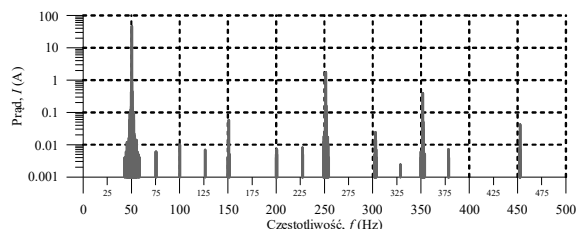
Rys. 13. Widma częstotliwościowe prądu dla asymetrycznej szczeliny powietrznej
