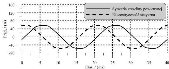
Rys. 5. Przebiegi czasowe prądu – symulacje komputerowe
