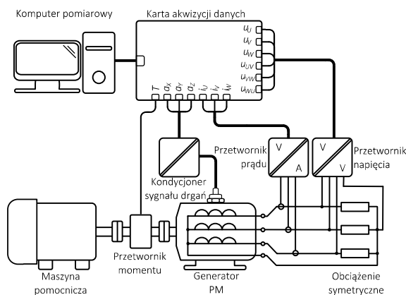
Rys. 9. Schemat pomiarowy
