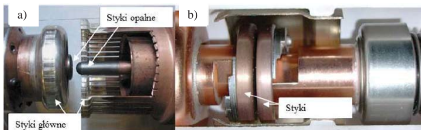
Rys. 3. Widok układów stykowych wyłącznika WN: gazowego – tulipanowego (a) i próżniowego – czołowego (b)
