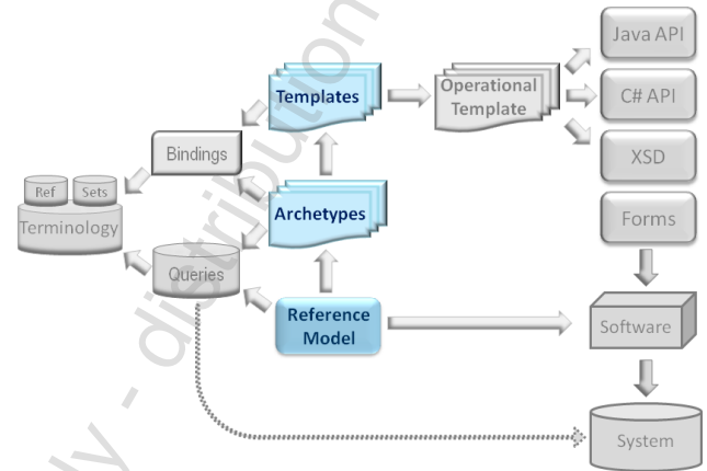
Rys. 3. Idea niezależnych modeli openEHR [21]
