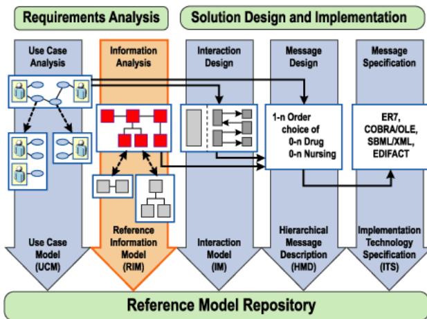
Rys. 2. Budowanie systemu wymiany informacji w HL7 [19]
