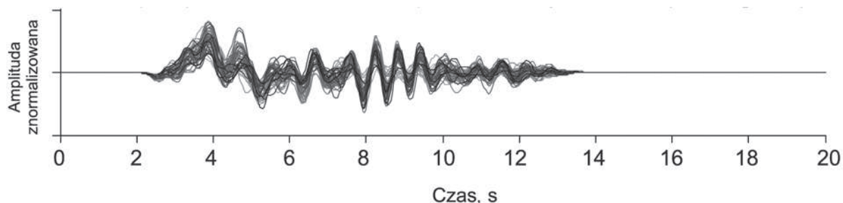
Rys. 6. Funkcja Greena obliczona z szumu sejsmicznego zarejestrowanego na terenie górnym w różnych dniach w warunkach prowadzonej eksploatacji
