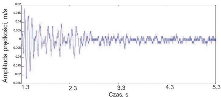
Rys. 8. Fale koda w rejestracji wstrząsu sejsmicznego z KWK Rydułtowy-Anna
