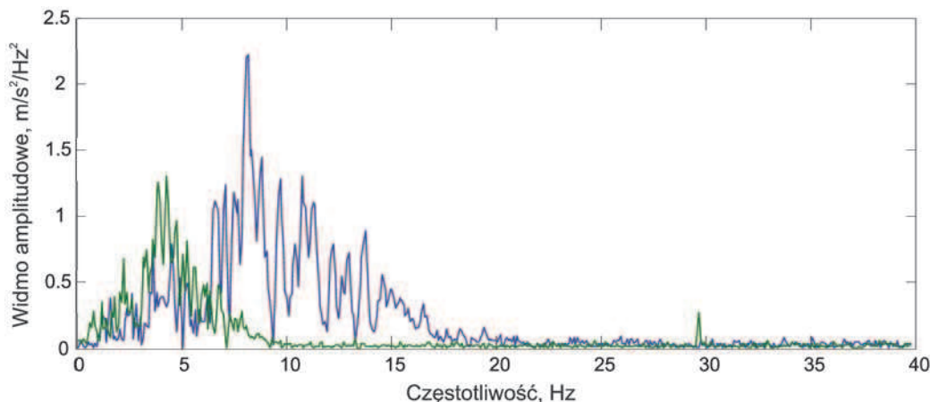
Rys 9. Widmo amplitudowe z zapisów pełnego (niebieska linia) i fali koda (zielona linia) rejestracji wstrząsu z kopalni Rydułtowy-Anna
