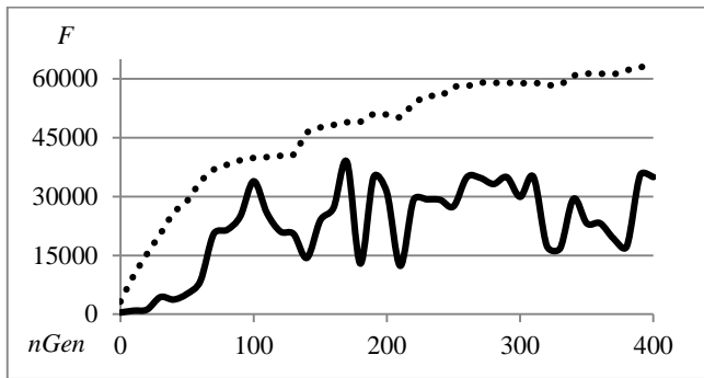
Rys. 12. Wyniki badań dla algorytmu IDA z wymianą najlepszego osobnika
