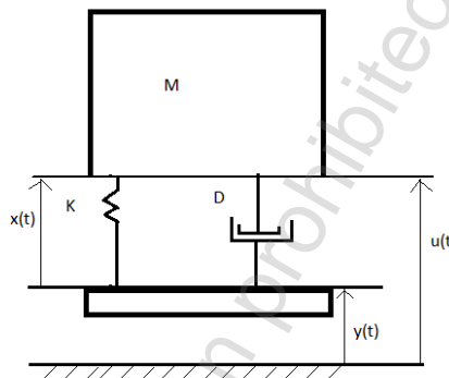
Rys. 3. Model mechaniczny sensora przyspieszenia [1]
