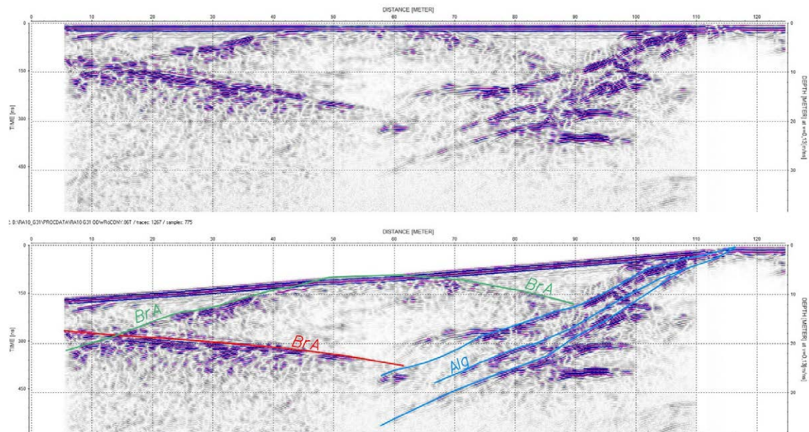
Ryc. 10. Echogram otworu Ra10 G-31 (a-echogram surowy, b-echogram z interpretacją), Alg-anhydryt górny, BrA-brekcja anhydrytowo-solna.
