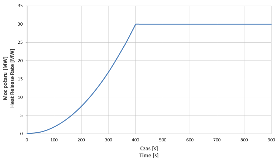
Ryc. 5. Przebieg przyjętej krzywej mocy pożaru dla 30MW Fig. 5. The course of the assumed fire curve for the value HRR of 30MW
