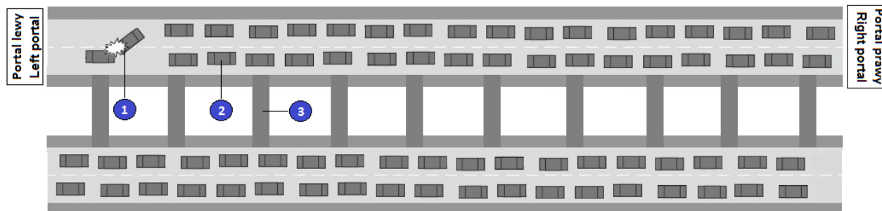
Ryc. 4. Lokalizacja pożaru przy wyjściu ewakuacyjnym (1) lokalizacja pożaru, (2) pojazdy w tunelu, (3) wyjścia ewakuacyjne Fig. 4. Fire location at an emergency exit (1) fire location, (2) vehicles in the tunnel, (3) emergency exits
