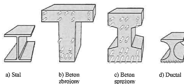
Rys. 1. Przekroje dźwigarów a) stal, b) żelbet c) beton sprężony d) Ductal
