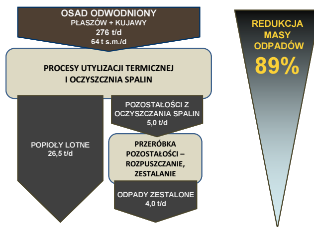
Rys. 3. Projektowy bilans masy odpadów w stacji termicznego unieszkodliwiania osadów oczyszczalni Kraków-Płaszów [7]
