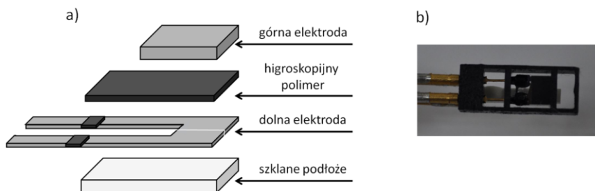
Rys. 3. Czujnik pojemnościowy; a) schemat budowy, b) zdjęcie czujnika [13]
