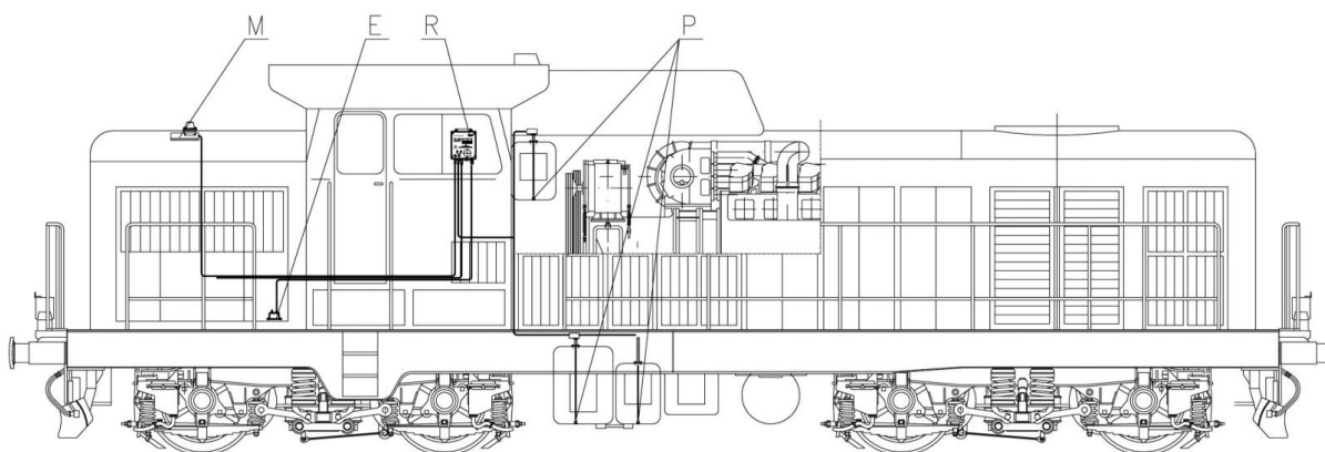
Rys. 3.3. Układ monitoringu masowego strumienia paliwa [16]: R – rejestrator CL400, P – hydrostatyczne sondy poziomu paliwa CL411, E – miernik energii elektrycznej, M – moduł telemetryczny GPRS/GPS i antena
