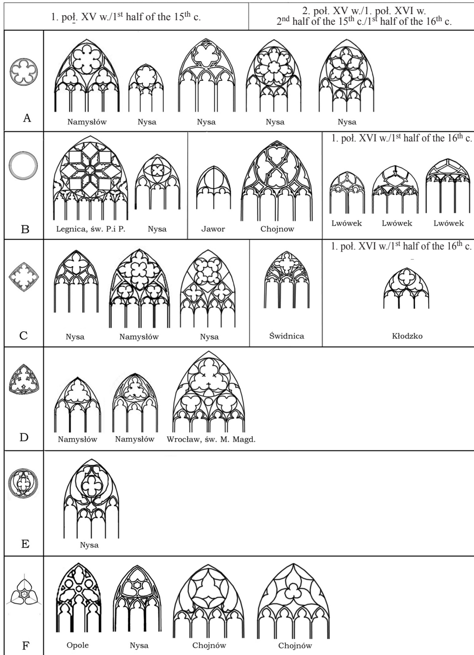
Il. 6. Maswerki o kompozycji centralnej (oprac. H. Golasz-Szołomicka)
