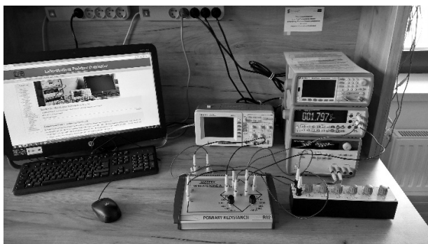
Rys. 3. Stanowisko laboratoryjne
