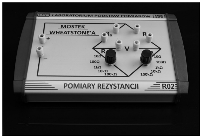
Rys. 2. Moduł pomiarowy
