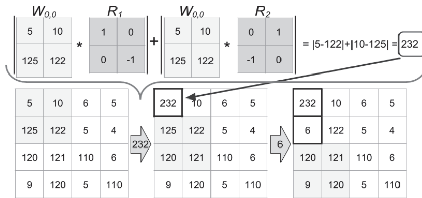
Rys. 2. Graficzna reprezentacja wykrywania krawędzi przy użyciu operatora krzyżowego Roberta
