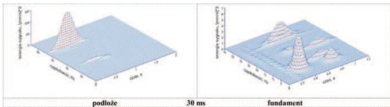
Rys. 17. Analiza MP drgań podłoża i fundamentu wzbudzanych milisekundowym odpaleniem ładunków MW z opóźnieniem 30 ms Fig. 17. MP analysis of the ground and structure foundation vibrations induced by millisecond blasting works – 30 ms time delay
