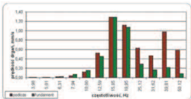
Rys. 14. Interakcja układu budynek-podłoże – kopalnia dolomitu – seria dwuszeregowa (17 ms i 67 ms)
