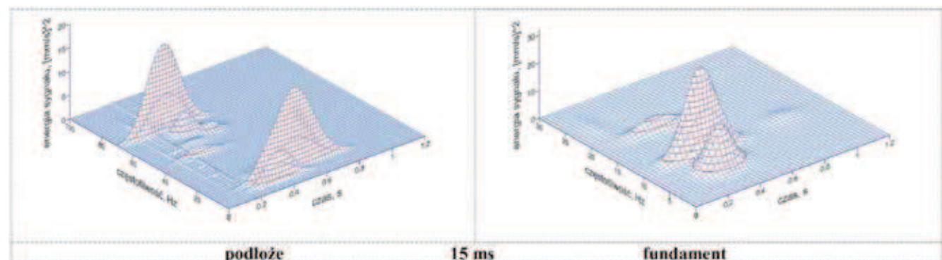
Rys.16. Analiza MP drgań podłoża i fundamentu wzbudzanych milisekundowym odpalaniem ładunków MW z opóźnieniem 15 ms
