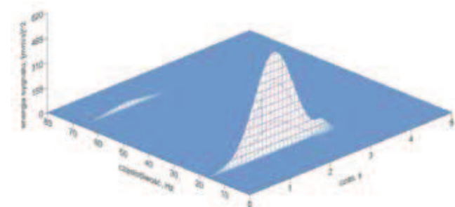
Rys. 9. Analiza czasowo-częstotliwościowa MP dla sejsmogramu z rysunku 6
