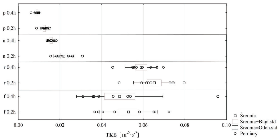
Rysunek 4. Wielkość turbulენტnej energii kinetycznej w poszczególnych lokalizacjach pomiarowych (p-ploso, n-nurt, r-bystrze, f-rwący nurt)
