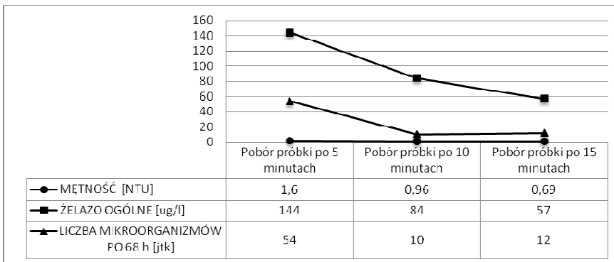
Rys. 2. Wykres zmienności parametrów wody pobieranej na węzle hydrantowym
