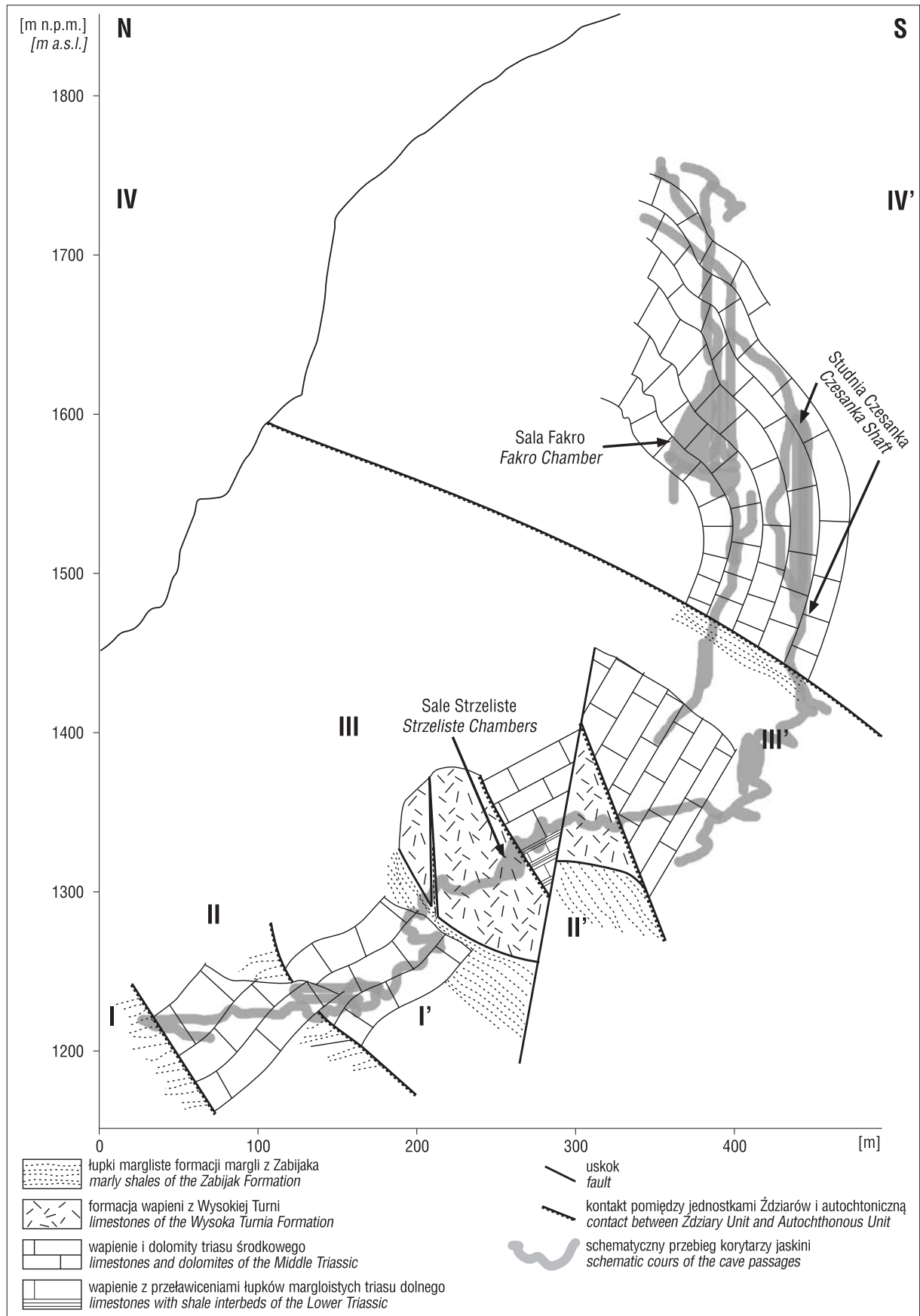
Ryc. 4. Przekroje geologiczne przez Jaskinię Małą w Mułowej (Szczygieł, 2013); dane geologiczne nie są zrzutowane na jedną płaszczyznę, a ich lokalizacja odpowiada dokładnie liniom wyznaczonym na rycinie 2
