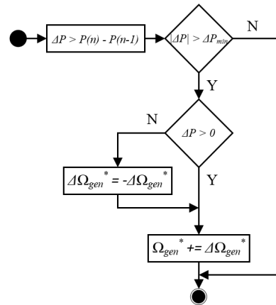
Rys. 10. Algorytm inkrementalnego śledzenia maksymalnego punktu mocy
