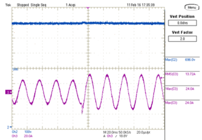
Rys. 15. Odpowiedź prądu fazowego generatora I_{su} i napięcia obwodu pośredniczącego U_{dc} na skokową zmianę momentu obciążenia T_m
