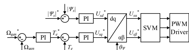
Rys. 7. Schemat blokowy metody bezpośredniego sterowania momentem DTC-SVM
