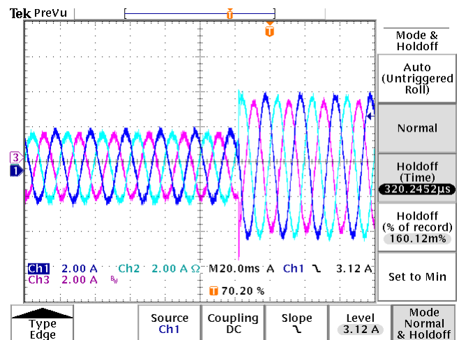
Rys. 14. Odpowiedź skokowa prądu sieci I_g
