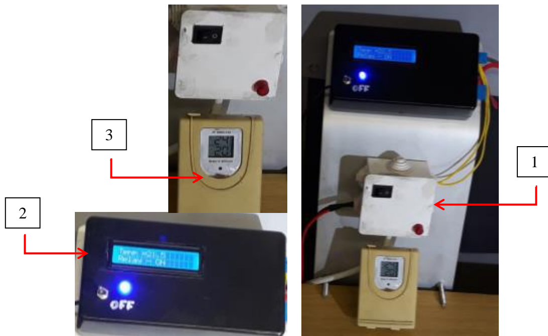
Rys. 3.4. Układ kontrolno-regulacyjny temperatury paliwa. 1 – termostat, 2 – regulator płyty grzewczej, 3 – rejestrator temperatury oraz wilgotności powietrza.
