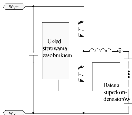
Rys. 8. Struktura układu zasobnika
