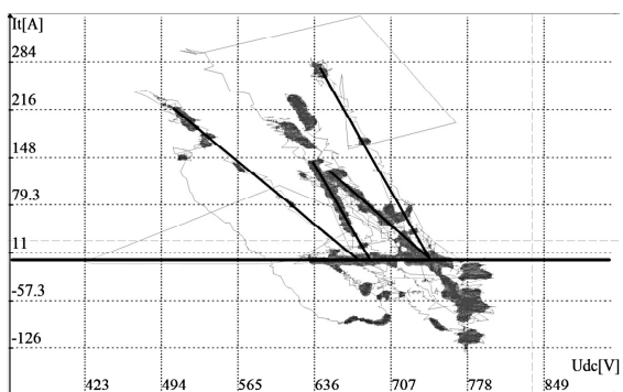
Rys. 4. Trajektorie z wyselekcjonowanymi obszarami o większym prawdopodobieństwie występowania pomiarów rejestrowanych ze stałym okresem impulsowania i naniesionymi liniami pozwalającymi na wyodrębnienie parametrów sieci
