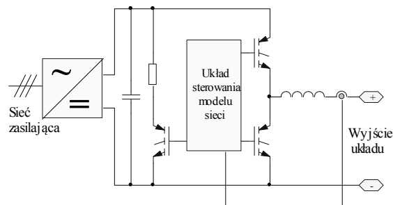
Rys. 6. Struktura modelu toru zasilania
