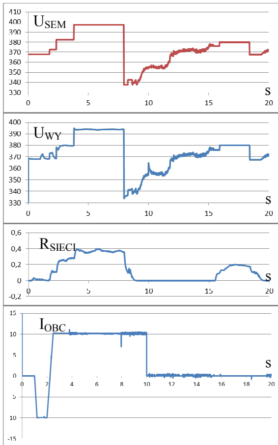
Rys. 7. Przebiegi zadanej napięcia zastępczego źródła U_{SEM} , napięcia wyjściowego układu U_{WY} , zadanej rezystancji sieci R_{SIECI} i prądu wyjściowego I_{WY}
