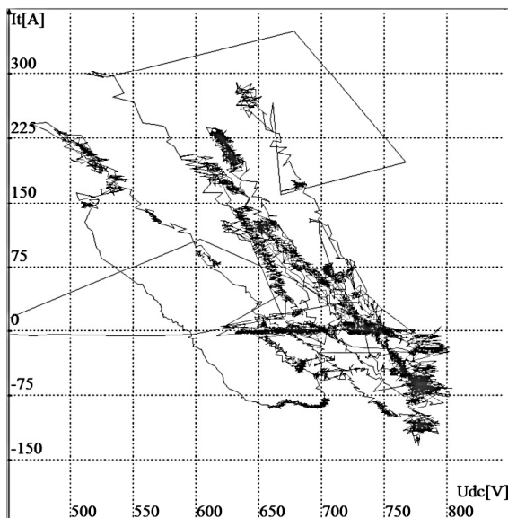
Rys. 3. Trajektorie prądowo-napięciowe napędu zarejestrowane podczas typowej jazdy ulicznej tramwaju
