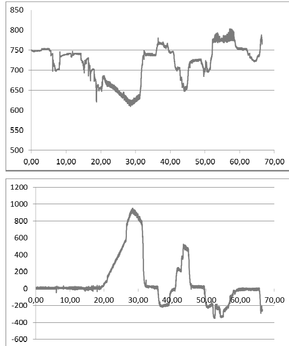
Rys. 2. Przykładowy przebieg napięcia sieci i pobieranego przez pojazd prądu
