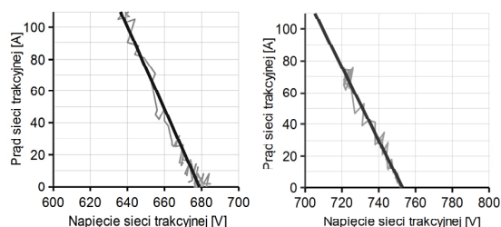
Rys. 5. Interpolacja liniowa trajektorii prądowo-napięciowej wykorzystana do wyznaczenia rezystancji szeregowej i napięcia sieci trakcyjnej
