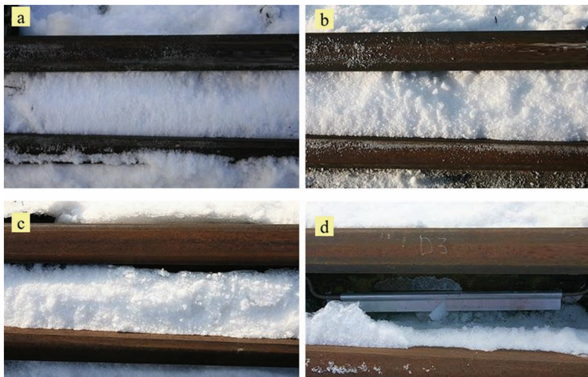
Rys. 7. Porównanie skuteczności wytapiania śniegu przez grzejniki standardowe i grzejniki bezстыkowe z radiatorem aluminiowym. Pomiar w warunkach bez opadów atmosferycznych i wiatru, temperatura otoczenia -24^{\circ}\text{C} ; a) grzejnik standardowy przed rozpoczęciem grzania, b) grzejnik bezстыkowy z radiatorem przed rozpoczęciem grzania, c) grzejnik standardowy po 4 godzinach grzania, d) grzejnik bezстыkowy z radiatorem po 4 godzinach grzania [fot. D. Brodowski]
