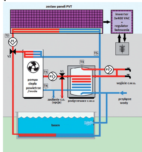
Rys. 5. Schemat instalacji ciepłowniczej dla domu jednorodzinnego wykorzystującej powietrzną pompę ciepła z wymiennikiem zasilanym z wodnych hybrydowych paneli fotowoltaicznych PVT Fig. 5. Heating installation diagram for a single-family house using an air heat pump with a heat exchanger powered by water hybrid PVT panels
