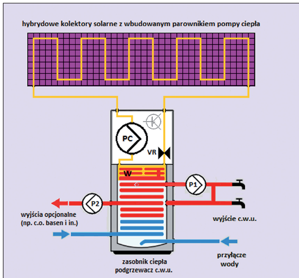
Rys. 8. Schemat instalacji grzewczej z udziałem fotowoltaicznej / termicznej pompy ciepła PVT-HP zespolonej z magazynem ciepła Fig. 8. Diagram of a heating installation with a PVT-HP combined solar thermal / heat pump combined with a heat storage
