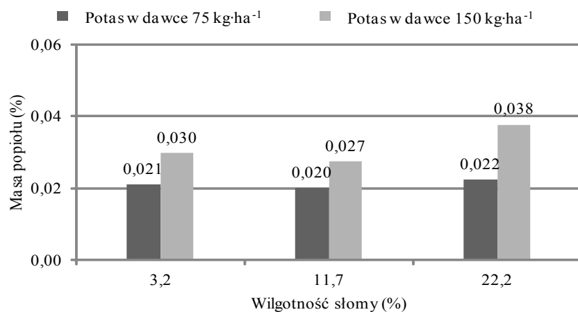
Rysunek 3. Średnia masa popiołu pozostałego po spaleniu próbki paliwa wytworzonego ze słomy orkiszu pszennego
