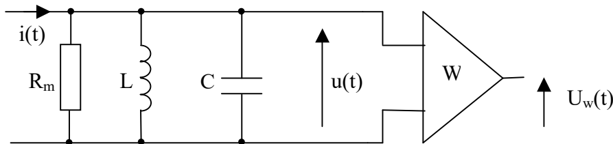
Rys. 1.3.3. Schemat zastępczy impedancji pomiarowej Z_m ze wzmacniaczem W [6]
