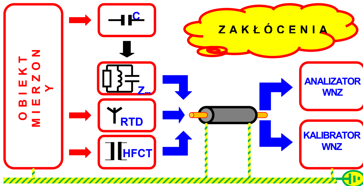
Rys. 1.3.7. Poglądowy schemat elektrycznego toru pomiarowego wyładowań niepełnych [12]
