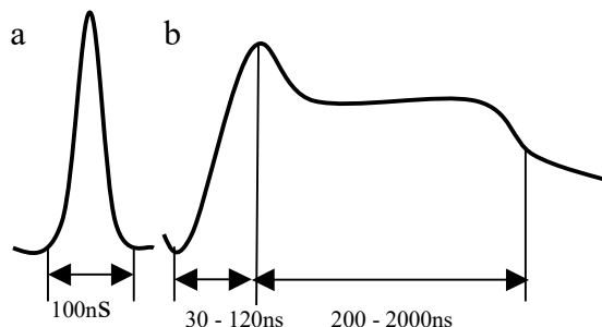
Rys. 1.3.6. Kształt oscylogramów prądów wnz [12, 26, 27, 28]: a – typowy (trójkątny) we wtrącinie, b – we wtrącinie o dużej średnicy (>5mm) po czasie przyłożenia napięcia >30min
