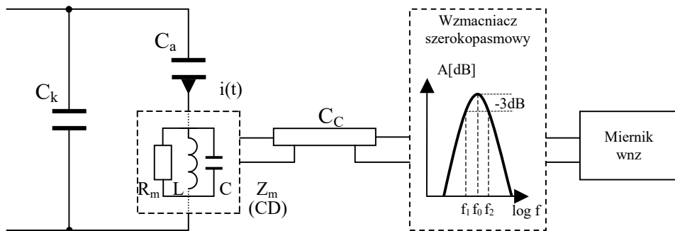
Rys. 1.3.2. Schemat układu pomiarowego w systemie szerokopasmowym [26]
