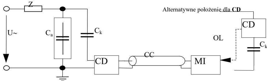
Rys. 1.3.1.a. Układ bezpośredni z szeregowym kondensatorem sprzęgającym [34]
