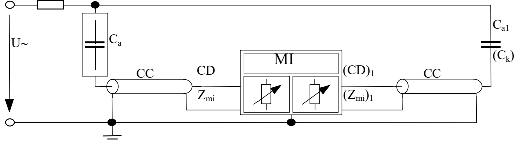
Rys. 1.3.1.c. Układ mostkowy [34]
