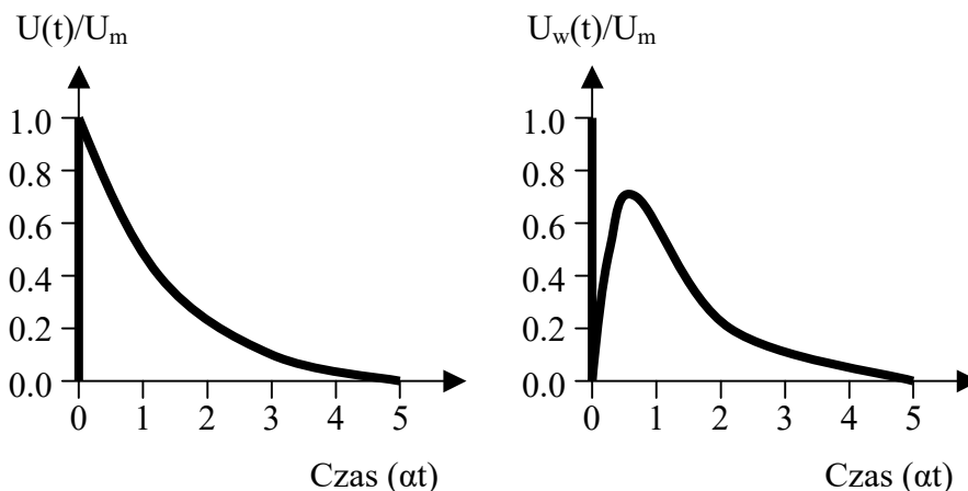
Rys. 1.3.4. Napięcie na wejściu wzmacniacza (a) i na wyjściu (b) – L=0 , \tau_w=0,3/a [6]
