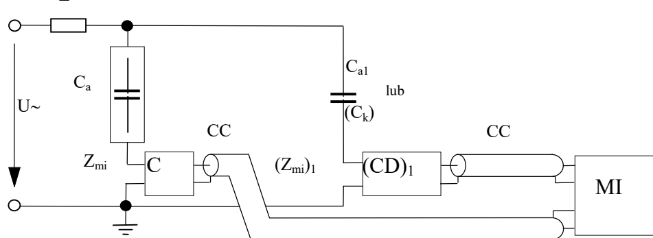
Rys. 1.3.1. d. Układ z detekcją polaryzacji [34]
