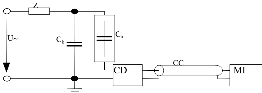
Rys. 1.3.1.b. Układ bezpośredni z szeregowo połączonym obiektem [34]
