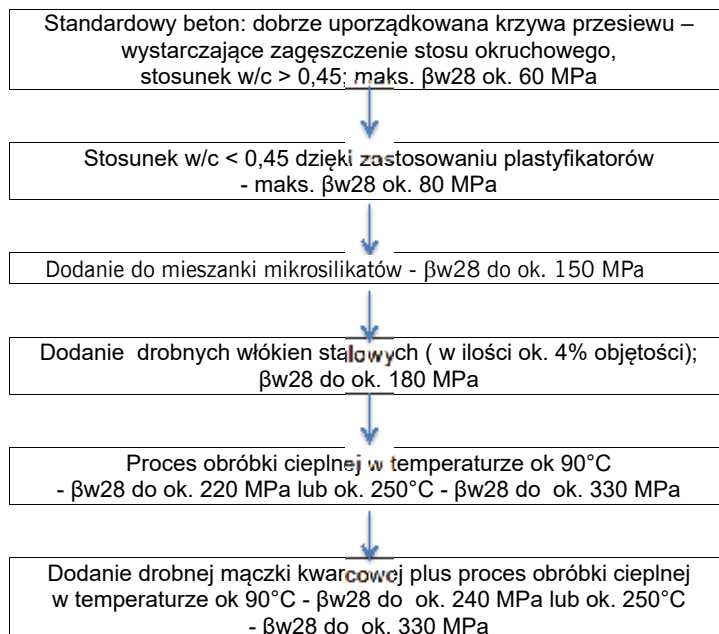
1. Kolejne kroki w rozwoju technologicznym mające na celu podwyższenie wytrzymałości betonu na ściskanie
