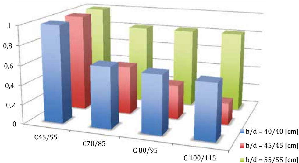
Rys. 2. Możliwość obniżenia stopnia zbrojenia w przypadku stosowania betonów wyższych klas względem słupów obiektów wielokondygnacyjnych z betonu C45/55 [4]
