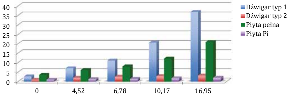
Rys. 4. Procentowy wzrost nośności elementów prefabrykowanych wg rysunku 5 wykonanych z betonu wysokowytrzymałego C100/115 względem elementów o tym samym przekroju oraz ilości stali sprężającej z betonu C50/60 [4]
