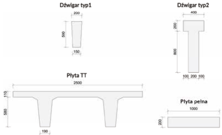
Rys. 3. Typowe przekroje porównawcze prefabrykatów
