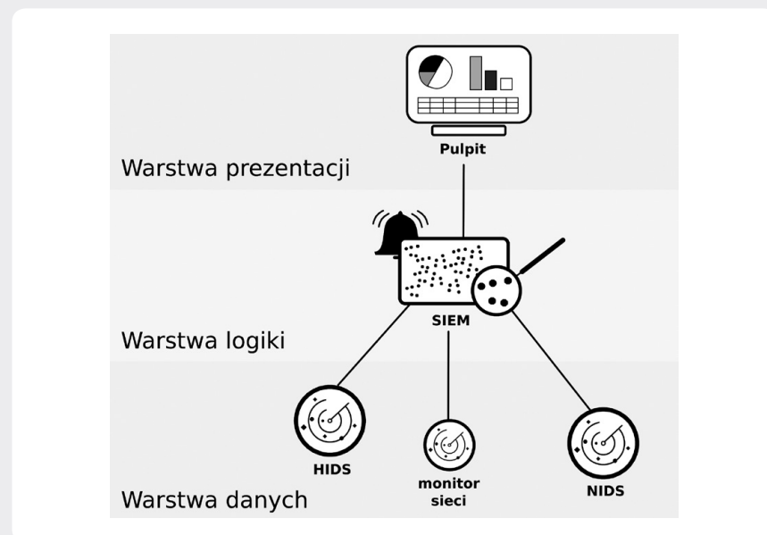
Rys. 2. Trójpoziomowa architektura SAN
