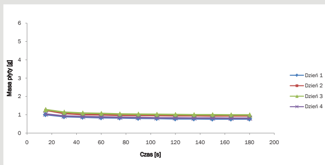
Rys. 6. Wyniki testu obciekania masy lelej SiC bez dodatku PVAL 47-88
