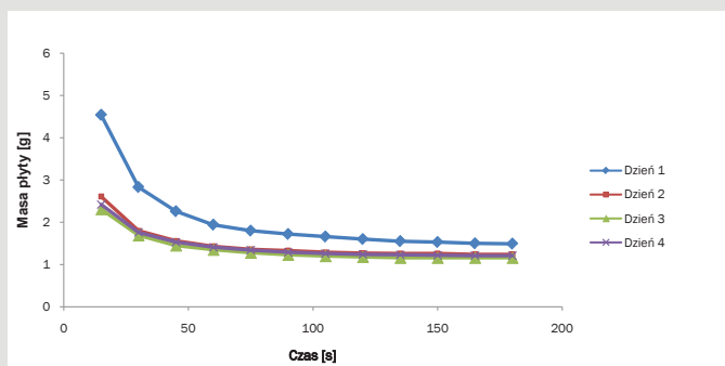
Rys. 8. Wyniki testu obciekania masy lelej SiC z dodatkiem 10% wag. PVAL 47-88
