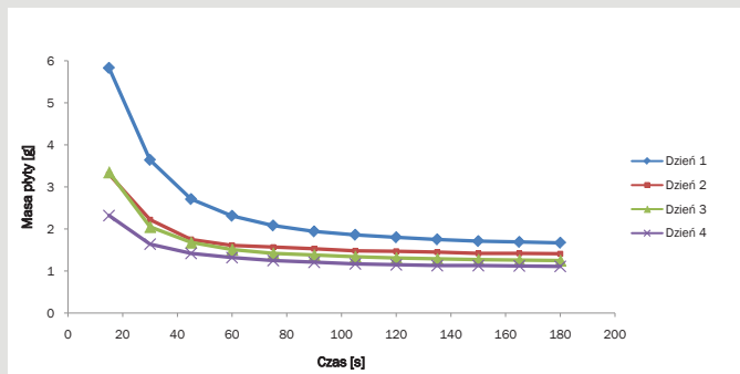
Rys. 9. Wyniki testu obciekania masy lelej SiC z dodatkiem 15% wag. PVAL 47-88
