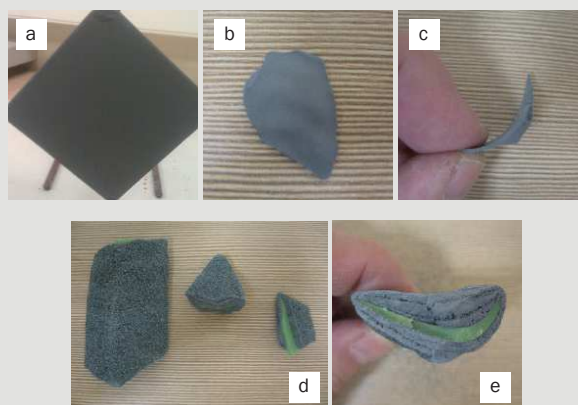
Rys. 10. Ocena adhezji masy formierskiej z 6% wag. udziałem PVAL do: (a) płyty mosiężnej; (b-c) modelu woskowego fragmentu łopatki silnika lotniczego (tzw. warstwa przymodelowa bez posypki); (d-e) trzech warstw wraz z posypkami.
