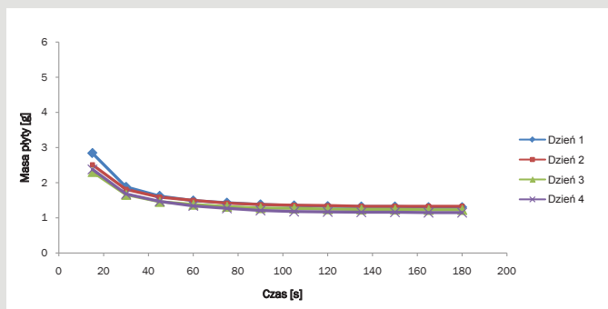
Rys. 7. Wyniki testu obciekania masy lelej SiC z dodatkiem 6% wag. PVAL 47-88
