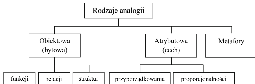
Rys. 3. Klasyfikacja analogii.
