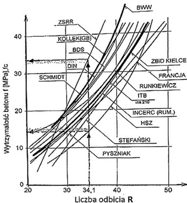
Rys. 2. Przykładowe zależności empiryczne f_c - R dla sklerometrów Schmidta typu N (dla różnych betonów w różnych krajach)
