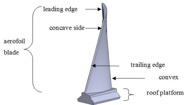
Fig. 1. Blade elements
