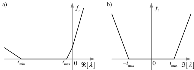
Rys. 3. Funkcje kary dla a) części rzeczywistej biegunu oraz b) części urojonej
