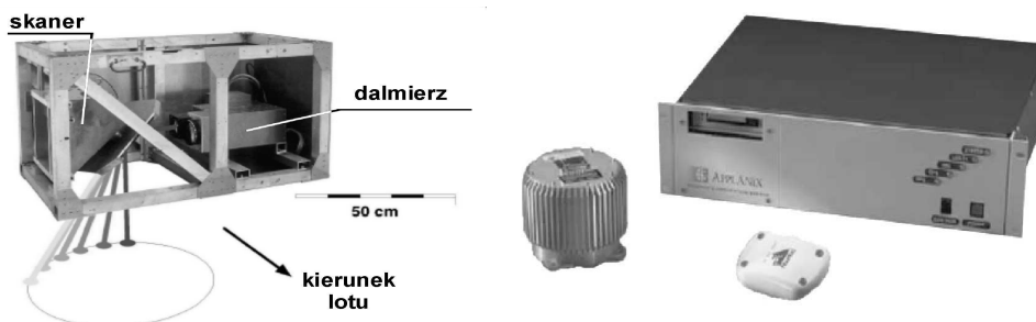
Rys. 1. Skaniny laserowe ScaLARS (po lewej) i Applanix POS/AV 510 (po prawej)
