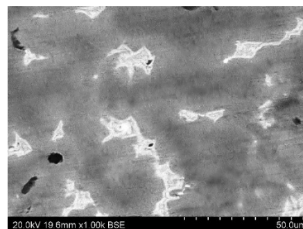
Fig. 10. Microstructure of the axe (NG25)
