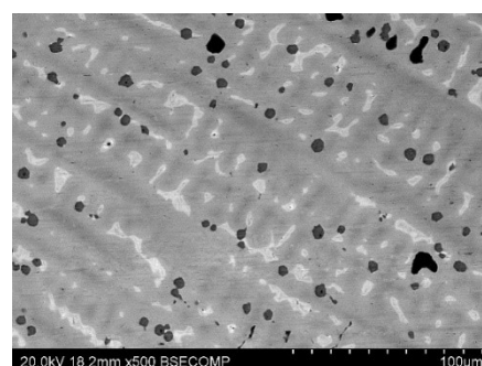
Fig. 11. Microstructure of the axe (NG21)
