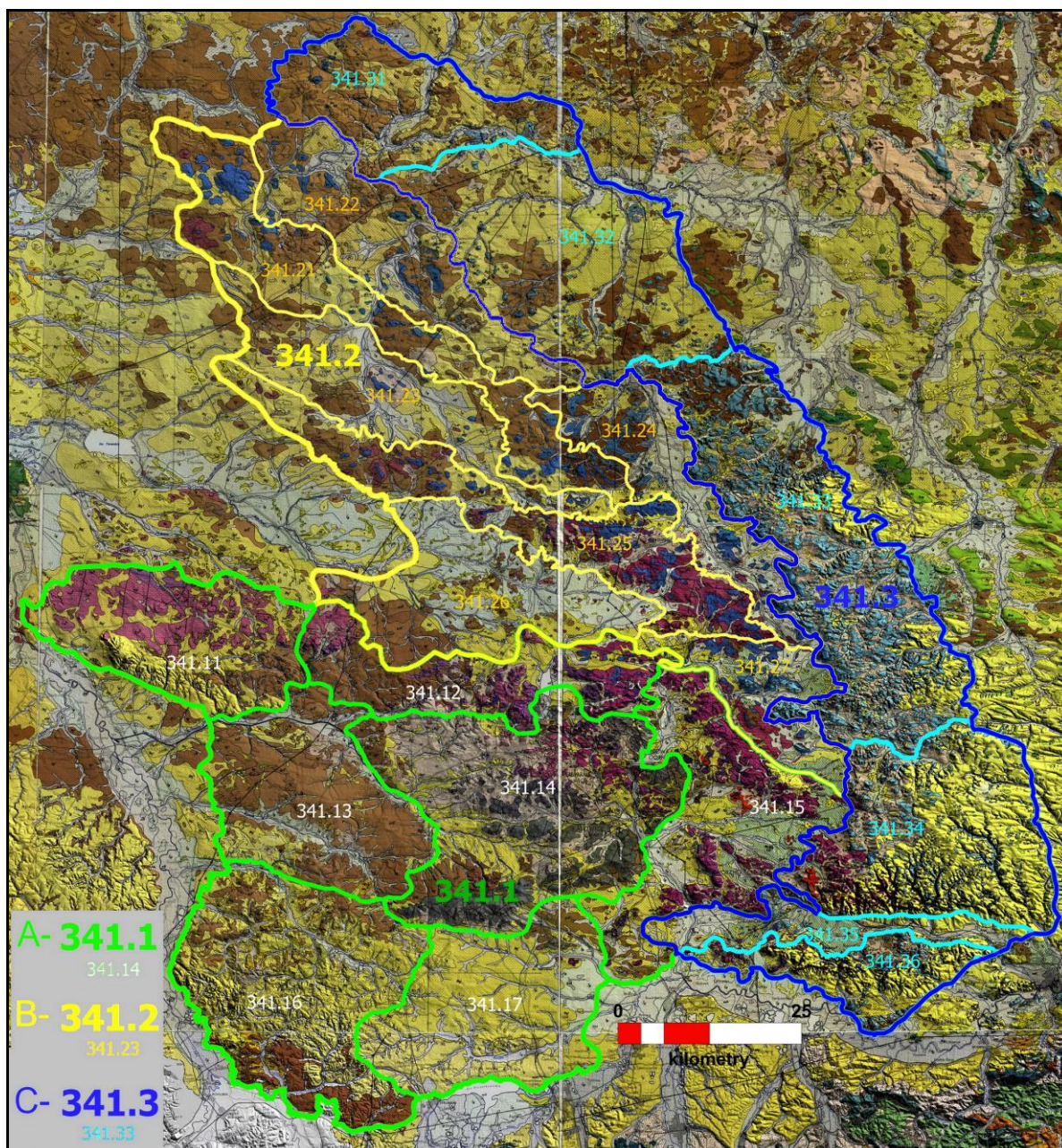
Ryc. 5. Propozycja korekty granic podprowincji Wyżyny Śląsko-Krakowskiej i makroregionów: A – 341.1 Wyżyna Śląska, B – 341.2 Wyżyna Woźnicko-Zawierciańska, C – 341.3 Wyżyna Krakowsko-Wieluńska) – na tle mapy geologicznej Polski. Źródło: opracowanie własne na podstawie; MgP – 1:200 000 A, PIG-PIB, ark. 71 – Bielsko-Biała, 70 – Cieszyn, 65 – Kraków, 64 – Gliwice, 65 – Kluczbork, 57 – Częstochowa, dane do NMT z CODGiK; ( http://mapy.geoportal.gov.pl/wss/service/ATOM/httpauth/atom/CODGIK_NMT100 ).
