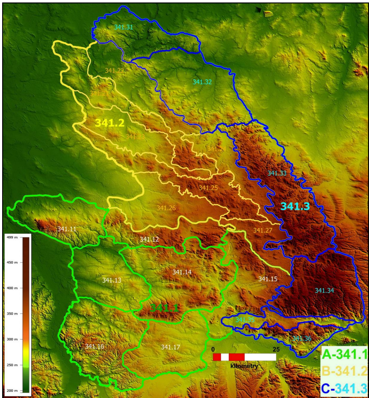
Ryc. 4. Propozycja podziału podprowincji Wyżyny Śląsko-Krakowskiej i makroregionów: A – 341.1 Wyżyna Śląska, B – 341.2 Wyżyna Woźnicko-Zawierciańska, C – 341.3 Wyżyna Krakowsko-Wieluńska. Kompozycja na tle NMT.
