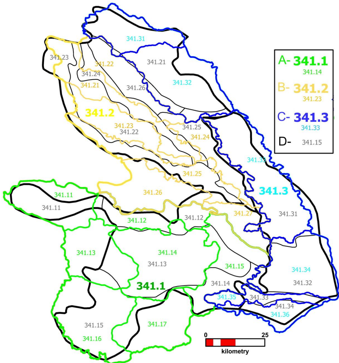
Ryc. 2. Zakres różnic w proponowanym podziale podprovincji Wyżyny Śląsko-Krakowskiej: A – 341.1 Wyżyna Śląska, B – 341.2 Wyżyna Woźnicko – Zawierciańska, C – 341.3 Wyżyna Krakowsko-Wieluńska (mezoregiony i makroregiony) D – na tle podziału wg. J. Kondrackiego. Źródło: Regiony fizycznogeograficzne według J. Kondrackiego i A. Richlinga, mapa ark. 53.3, Atlas Rzeczypospolitej Polskiej (1993-1997, GGK).
