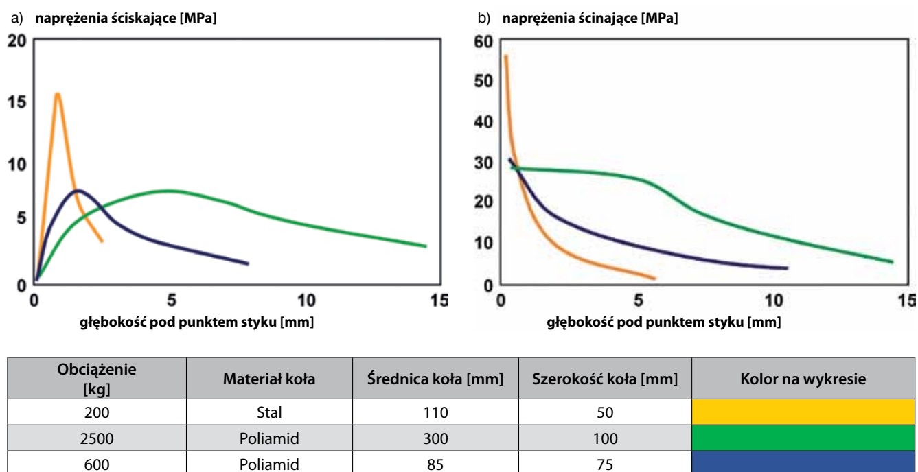
Rys. 2. Naprężenia: a) ściskające wywołane dociskiem koła, b) ścinające na posadzce betonowej w zależności od rodzaju ogumienia pojazdów, według [34]
