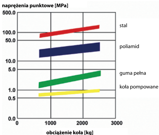
Rys. 1. Naprężenia kontaktowe wywołane dociskiem koła na posadzce betonowej w zależności od rodzaju ogumienia pojazdów, według [34]
