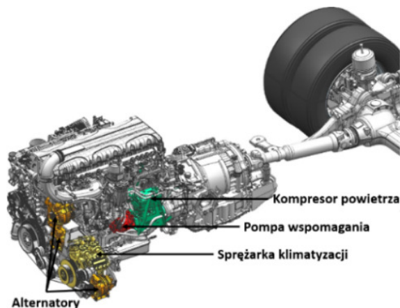
Rys. 5. Akcesoria zasilane z silnika spalinowego[1]
