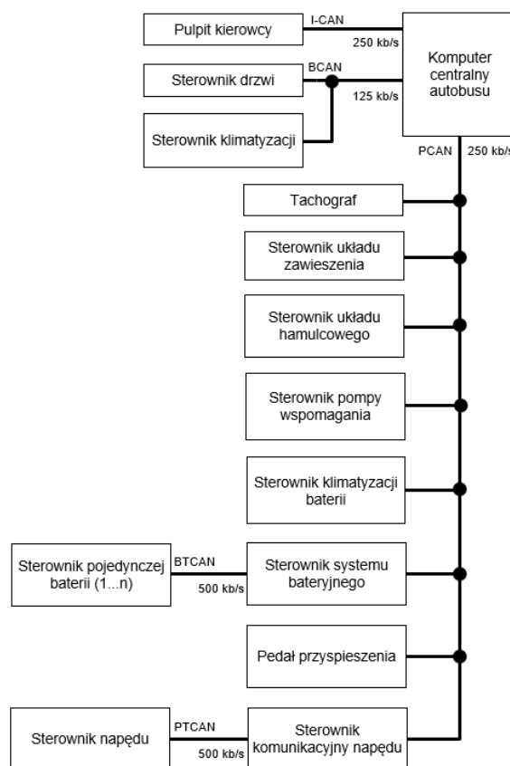
Rys. 9. Architektura magistrali komunikacyjnej CAN systemu nadzorczo-sterującego autobusu baterijnego[1]
