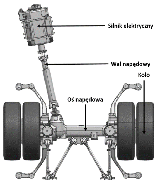
Rys. 7. Architektura systemu napędowego – napęd elektryczny[1]
