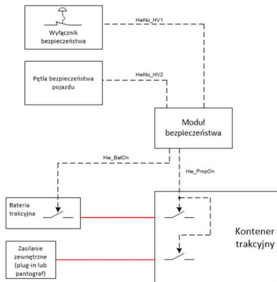
Rys. 10. Wylącznik awaryjny i pętla bezpieczeństwa [1]
