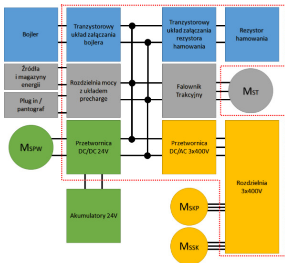
M ST – silnik trakcyjny M SPW – silnik pompy wspomaganie M SKP – silnik kompresora powietrza M SSK – silnik sprężarki klimatyzacji *** układ energoelektroniczny w autobusie baterijnym ■ obwód instalacji zasilanej napięciem 24V DC ■ obwód instalacji zasilanej napięciem 3x400V AC ■ układ napędowy według definicji klasycznej
