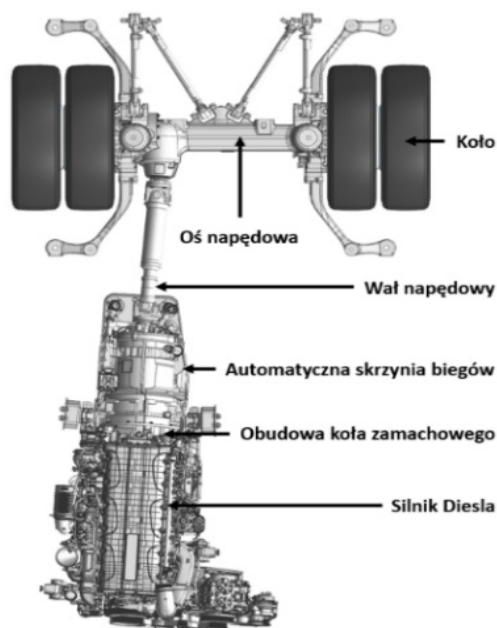
Rys. 4. Architektura systemu napędowego – napęd konwencjonalny [1]
