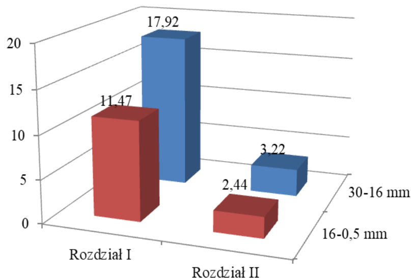
Rys. 3. Udziały frakcji <1,4 \text{ g/cm}^3 w produkcji odpadowym [4]
