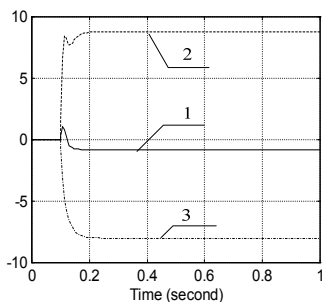
Rys. 14. Zarejestrowane przebiegi urojonej części spadków napięć w woltach: 1) na impedancji Z_1 , 2) na impedancji Z_2 , 3) na impedancji Z_3
