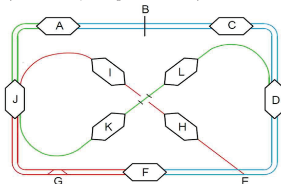
Rys. 1. Schemat ideowy wirtualnej sieci kolejowej tworzonej w ramach powstającego laboratorium inżynierii ruchu kolejowego na Wydziale Inżynierii Lądowej Politechniki Krakowskiej
