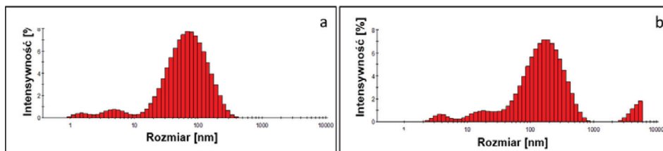
Rysunek 6. Rozkład wielkości nanocząstek złota otrzymanych metodą klasyczną wspomaganą mikrofalami o mocy 800 W: z cytrynianem trisodu (a) oraz z gumą arabską (b)
