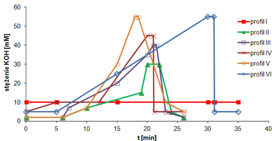
Rysunek 1. Profile stężeń eluentej: izokratyczny (stałe stężenie KOH = 10 mM – profil I) i gradientowe (profile II–VI).
