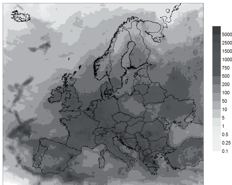
RYSUNEK 2. Depozycja azotu [ \text{mg}\cdot\text{m}^{-2} ] w 2012 roku w wyniku emisji ze źródeł w domenie obliczeniowej zlokalizowanych poza obszarem Polski (zob. objaśnienia w tekście, punkt 1)
