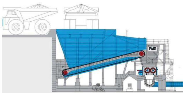
Rys. 4. Układ kruszenia bez wstępnego odsiewania z dozowaniem przenośnikiem stalowo-członowym firmy FAM [16]
