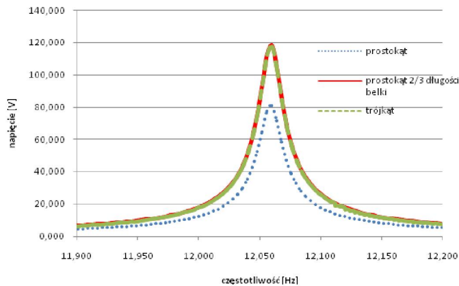
Rys. 4. Charakterystyki amplitudowo-częstotliwościowe generowanego napięcia, drgania w zakresie pierwszej częstotliwości rezonansowej Fig. 4. Amplitude-frequency characteristics of generated voltage, the first natural frequency vibrations
