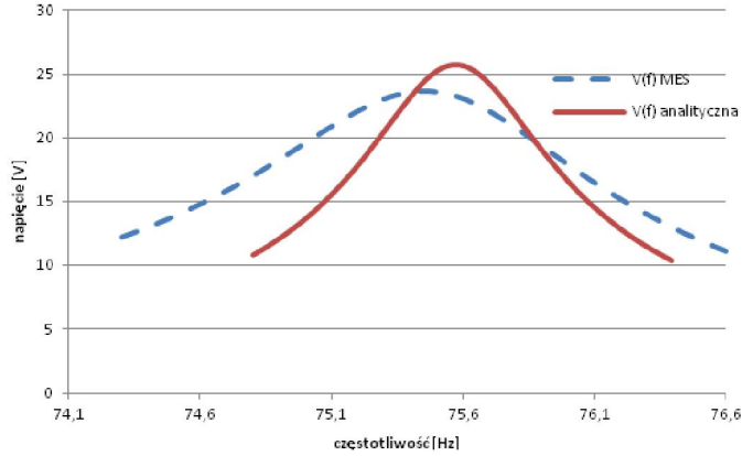
Rys. 7. Charakterystyki amplitudowo-częstotliwościowe generowanego napięcia, drgania w zakresie drugiej częstotliwości rezonansowej; porównanie wyników metody analitycznej i MES
