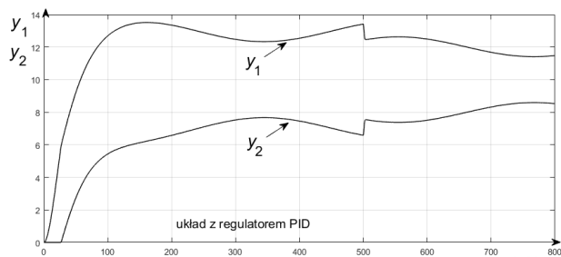
Rys. 14. Przebiegi wielkości regulowanych y_1 i y_2 dla zadanej różnicy temperatur - regulator PID
