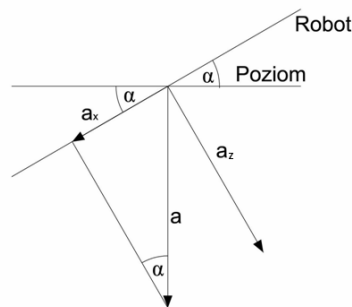
Rys. 2. Rozkład wektora przyspieszenia ziemskiego
