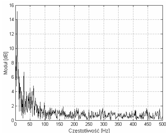
Rys. 3. Widmo sygnału bez filtracji
