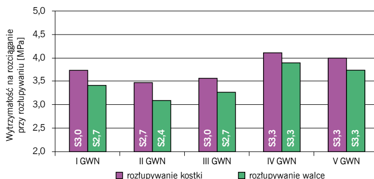
Rys. 3. Zestawienie średnich wytrzymałości na rozciąganie przy rozłupywaniu betonu stosowanego do górnej warstwy nawierzchni w zależności od rodzaju próbek do badań
